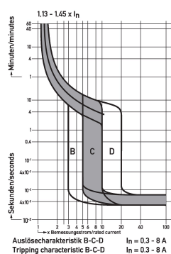
Diagramme Leitungsschutzschalter DLS 6h Bo6-3
