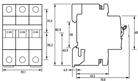
Maßzeichnung Leitungsschutzschalter DLS 6h Bo6-3
