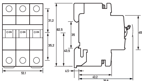
Maßzeichnung Leitungsschutzschalter DLS 6h C13-3
