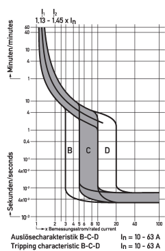
Diagramme Leitungsschutzschalter DLS 6h C13-3
