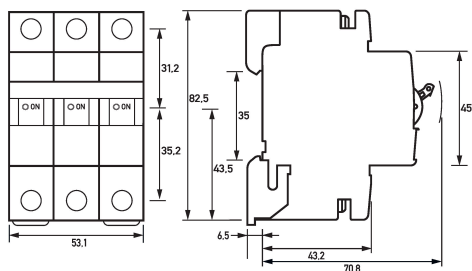
Maßzeichnung Leitungsschutzschalter DLS 6h Co6-3
