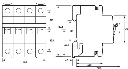
Maßzeichnung Leitungsschutzschalter DLS 6i B10-3+N
