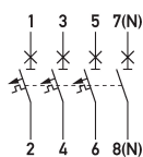
Schaltungsbeispiel Leitungsschutzschalter DLS 6i B10-3+N
