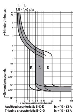
Diagramme Leitungsschutzschalter DLS 6i B16-4
