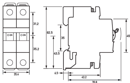
Maßzeichnung Leitungsschutzschalter DLS 6i B40-1+N
