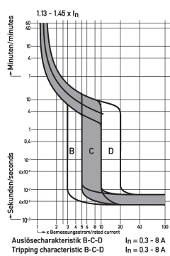
Diagramme Leitungsschutzschalter DLS 6i Bo6-1
