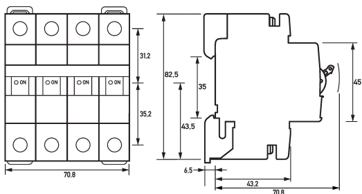
Maßzeichnung Leitungsschutzschalter DLS 6i Bo6-3+N
