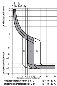
Diagramme Leitungsschutzschalter DLS 6i C10-3+N
