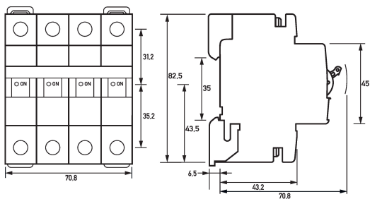
Maßzeichnung Leitungsschutzschalter DLS 6i C16-4
