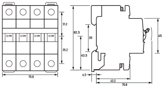
Maßzeichnung Leitungsschutzschalter DLS 6i C50-3+N
