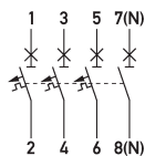
Schaltungsbeispiel Leitungsschutzschalter DLS 6i C50-3+N
