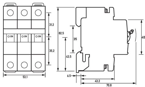
Maßzeichnung Leitungsschutzschalter DLS 6i Co6-3
