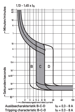
Diagramme Leitungsschutzschalter DLS 6i Co6-3
