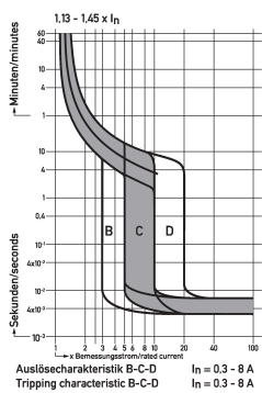
Diagramme Leitungsschutzschalter DLS 6i Co8-1+N
