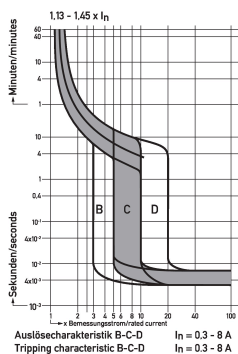
Diagramme Leitungsschutzschalter DLS 6i Co8-3+N
