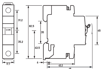
Maßzeichnung Leitungsschutzschalter DLS 6i D13-1
