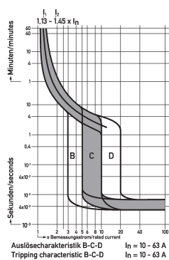
Diagramme Leitungsschutzschalter DLS 6i D16-3
