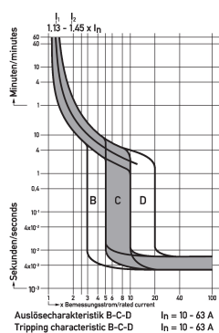
Diagramme Leitungsschutzschalter DLS 6i D25-3
