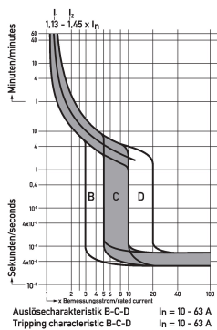
Diagramme Leitungsschutzschalter DLS 6i D50-3+N
