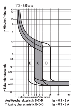
Diagramme Leitungsschutzschalter DLS 6i Do6-3
