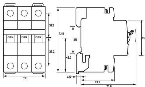
Maßzeichnung Leitungsschutzschalter DLS 6i Do6-3
