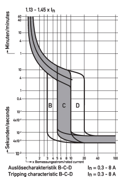
Diagramme Leitungsschutzschalter DLS 6i Do6-3+N
