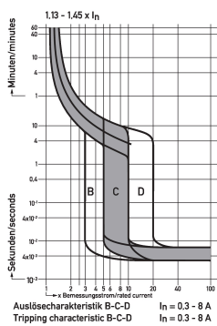
Diagramme Leitungsschutzschalter DLS 6i Do8-1+N
