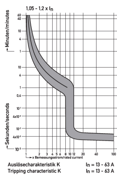
Diagramme Leitungsschutzschalter DLS 6i K20-4
