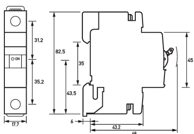
Maßzeichnung Leitungsschutzschalter DLS 6i K63-1
