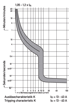
Diagramme Leitungsschutzschalter DLS 6i K63-3
