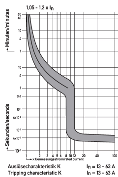
Diagramme Leitungsschutzschalter DLS 6i K63-4
