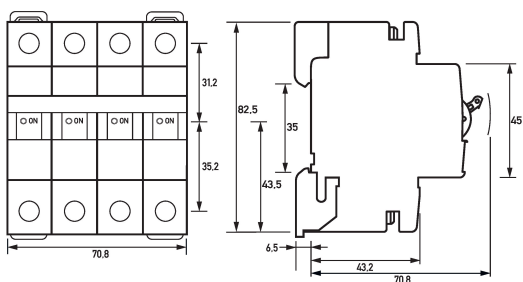
Maßzeichnung Leitungsschutzschalter DLS 6i Ko8-4
