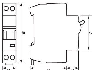
Maßzeichnung Leitungsschutzschalter ELS 3 C10/1+N
