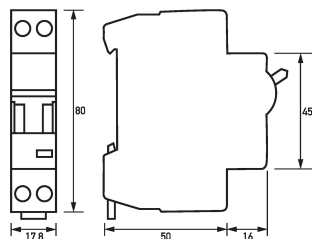
Maßzeichnung Leitungsschutzschalter ELS 3 C13/1+N
