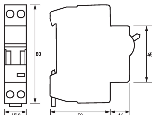
Maßzeichnung Leitungsschutzschalter ELS 3 Co2/1+N
