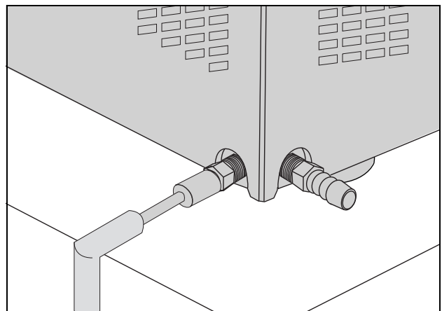
Afb. 9: Condensafvoer aansluiten
