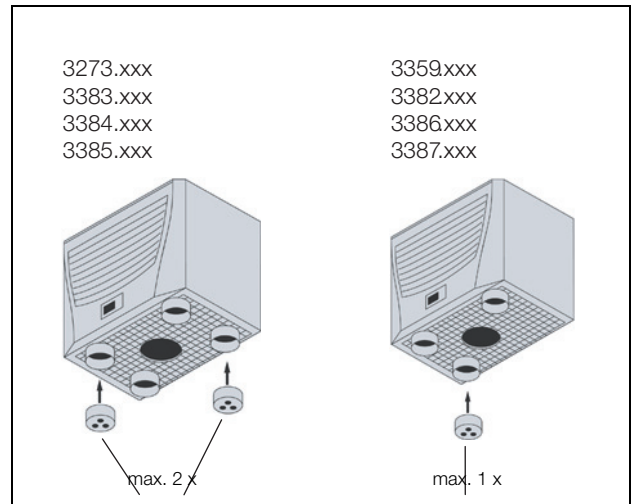
Afb. 5: Afsluitdoppen
