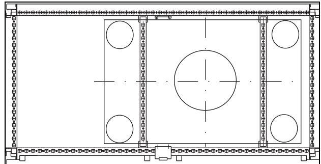
Afb. 8: Dakplaatversteviging bij TS 8 kast
