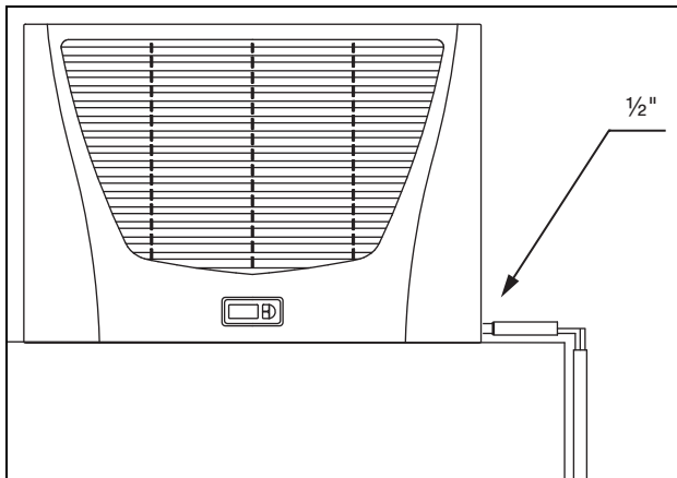
Afb. 10: Condensafvoer plaatsen
