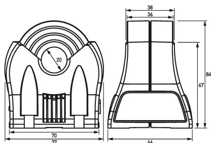
Maßzeichnung Differenzstromwandler DCT A-020
