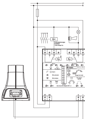
Schaltungsbeispiel Differenzstromwandler DCT A-020
