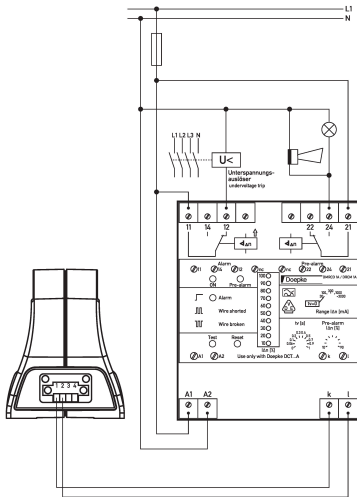
Schaltungsbeispiel Differenzstromwandler DCT A-105
