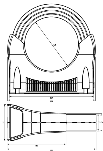
Maßzeichnung Differenzstromwandler DCT A-105
