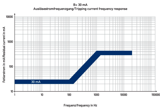
Diagramme Fehlerstromschutzschalter DFS 2 016-2/0,03-B+
