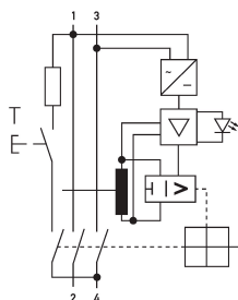
Schaltungsbeispiel Fehlerstromschutzschalter DFS 2 016-2/0,30-B+
