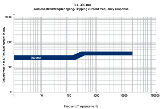
Diagramme Fehlerstromschutzschalter DFS 2 016-2/0,30-B+
