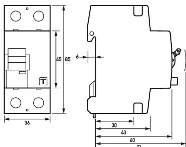
Maßzeichnung Fehlerstromschutzschalter DFS 2 016-2/0,30-B+
