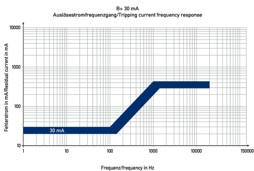
Diagramme Fehlerstromschutzschalter DFS 2 025-2/0,03-B+
