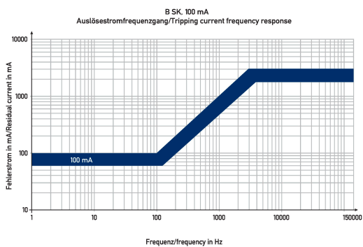
Diagramme Fehlerstromschutzschalter DFS 2 025-2/0,10-B SK
