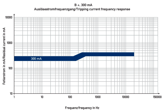
Diagramme Fehlerstromschutzschalter DFS 2 025-2/0,30-B+
