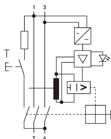
Schaltungsbeispiel Fehlerstromschutzschalter DFS 2 025-2/0,30-B+
