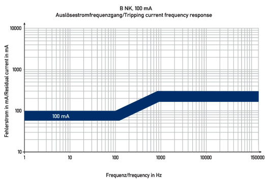
Diagramme Fehlerstromschutzschalter DFS 2 040-2/0,10-B NK
