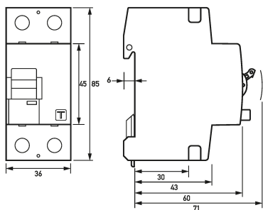
Maßzeichnung Fehlerstromschutzschalter DFS 2 040-2/0,10-B NK
