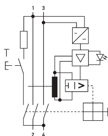
Schaltungsbeispiel Fehlerstromschutzschalter DFS 2 040-2/0,30-B+
