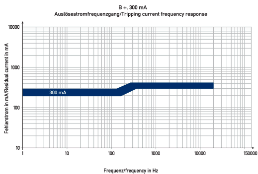
Diagramme Fehlerstromschutzschalter DFS 2 040-2/0,30-B+
