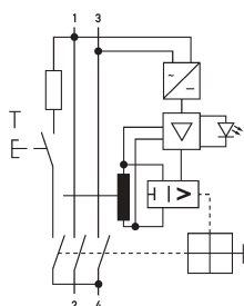
Schaltungsbeispiel Fehlerstromschutzschalter DFS 2 063-2/0,03-B+
