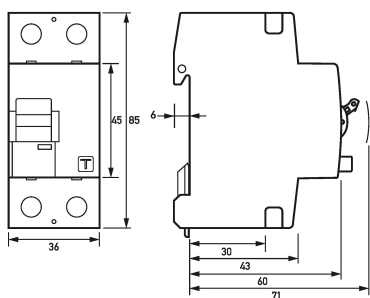
Maßzeichnung Fehlerstromschutzschalter DFS 2 063-2/0,10-B NK
