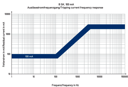
Diagramme Fehlerstromschutzschalter DFS 2 080-2/0,10-B SK
