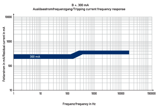
Diagramme Fehlerstromschutzschalter DFS 2 080-2/0,30-B+
