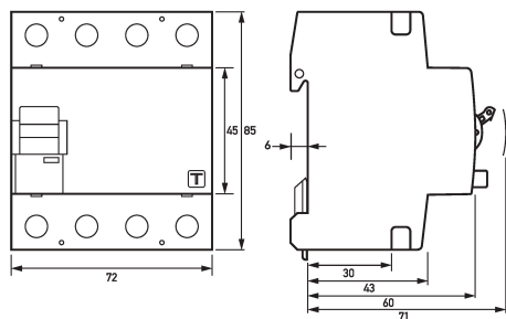
Maßzeichnung Fehlerstromschutzschalter DFS 4 016-4/0,30-B NK HD
