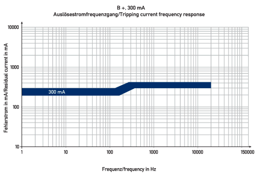
Kennlinie B+ 300 mA
