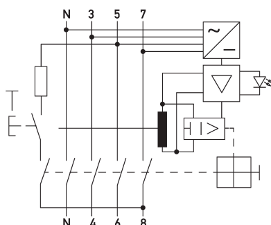
Schaltungsbeispiel Fehlerstromschutzschalter DFS 4 025-4/0,03-B SK MI HD
