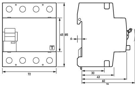
Maßzeichnung Fehlerstromschutzschalter DFS 4 025-4/0,03-B SK MI HD
