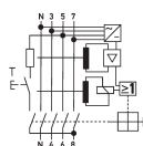
Schaltungsbeispiel Fehlerstromschutzschalter DFS 4 025-4/0,03-F EV HD
