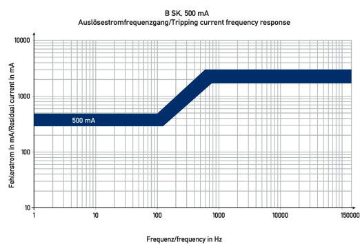
Diagramme Fehlerstromschutzschalter DFS 4 040-4/0,50-B SK HD
