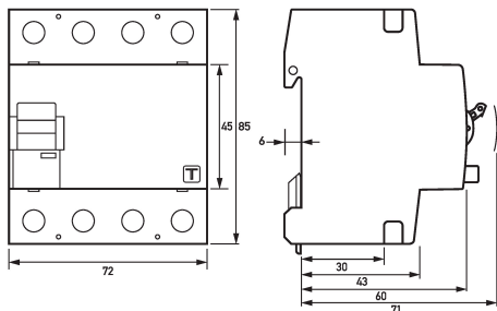
Maßzeichnung Fehlerstromschutzschalter DFS 4 063-4/0,50-B SK MI
