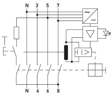
Schaltungsbeispiel Fehlerstromschutzschalter DFS 4 063-4/0,50-B SK MI
