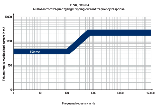
Diagramme Fehlerstromschutzschalter DFS 4 063-4/0,50-B SK MI
