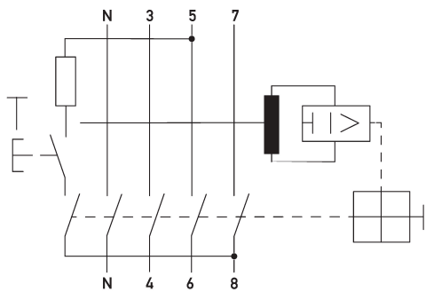
Schaltungsbeispiel Fehlerstromschutzschalter DFS 4 100-4/0,50-A HD
